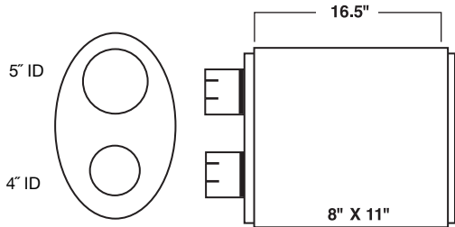
MODEL: CAT D4
