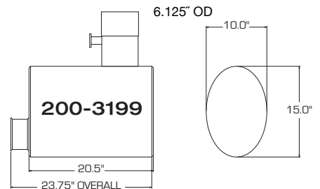
D8N, D8R DOZERS
