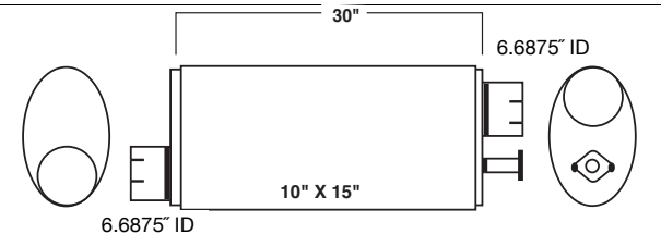
MODEL: CAT 988B 7W8445
