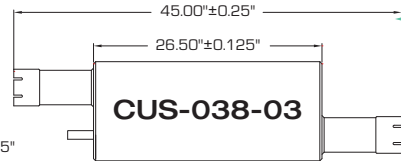
CUS-038-03 INTERNATIONAL 1175 END LOADER O.E# 680690
